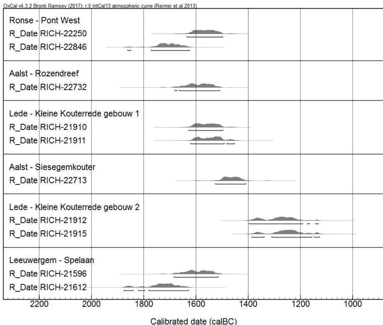
Fig. 8. Multiplot van de ^{14}\text{C} -dateringen.
