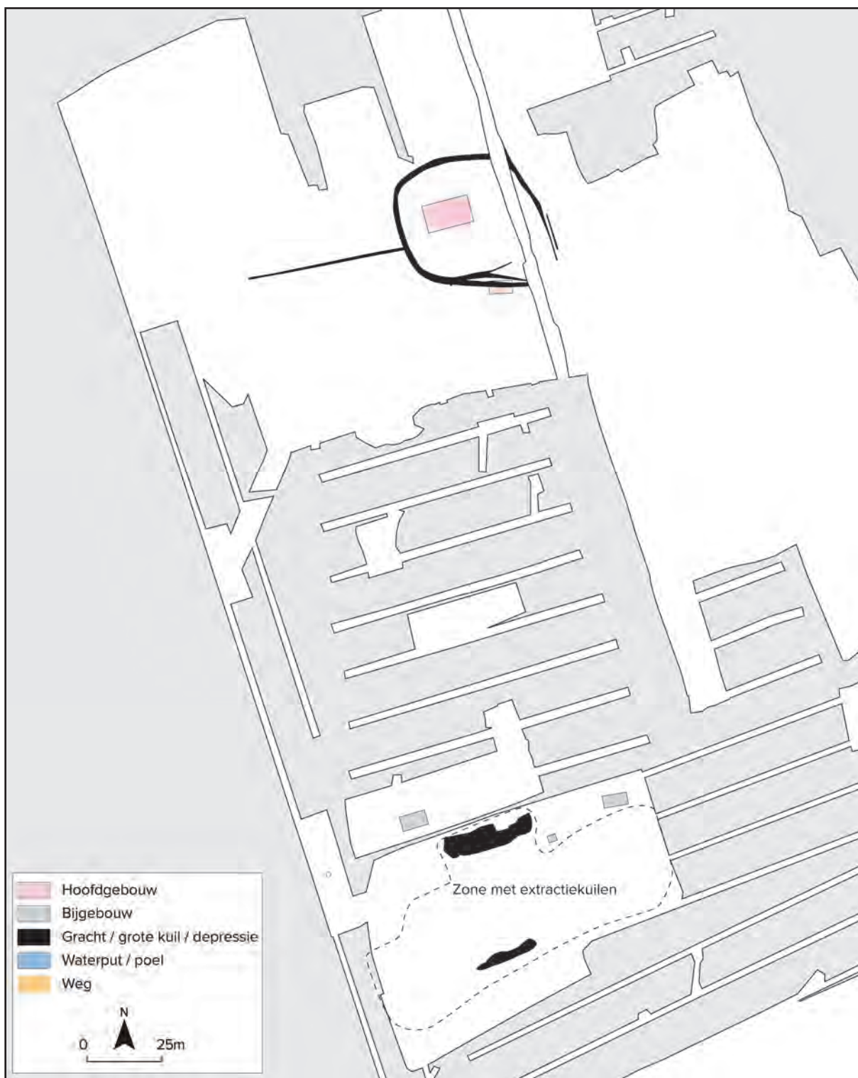
Fig. 2.9. Voorbeeld van een kleine, gebogen omgrachte nederzetting uit de 10de eeuw. Vereenvoudigd grondplan van de 10de-eeuwse fase op de site Ronse – Pont West.
